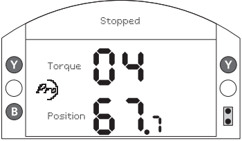
图 4.4.4 Torque (D) + Position 阀位 + 力矩数字显示
