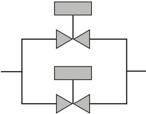
Fig 2. 1oo2 — 过程阀门旁路配置
