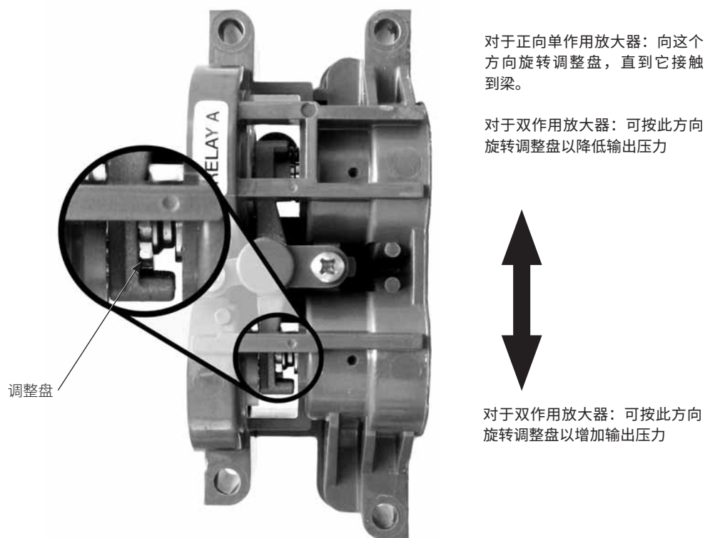
图 29. A 型放大器调整（为清晰起见，已拆除护套）
