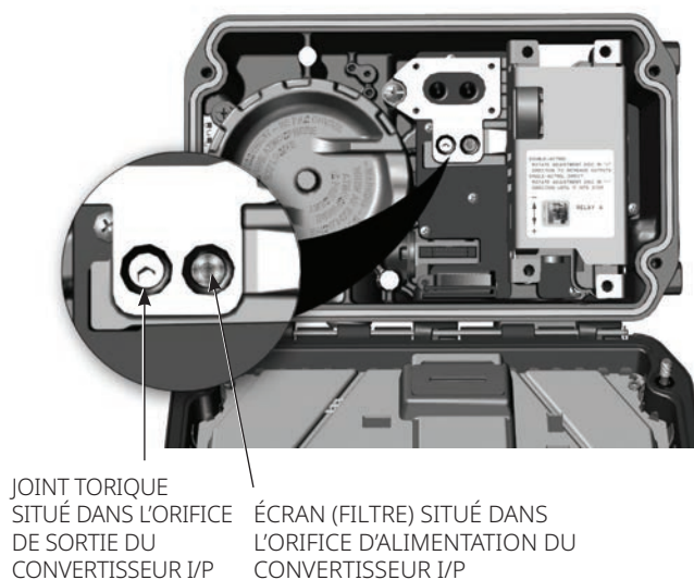
Figure 14. Emplacement du filtre I/P
