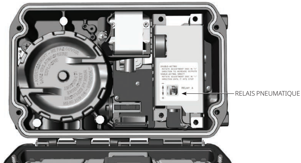
Figure 20. Emplacement du relais pneumatique
