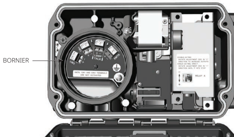
Figure 22. Emplacement du bornier
