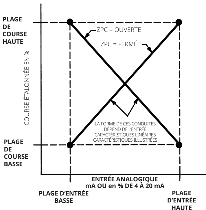
Figure 7. Relation entre la course étalonnée et l'entrée analogique
