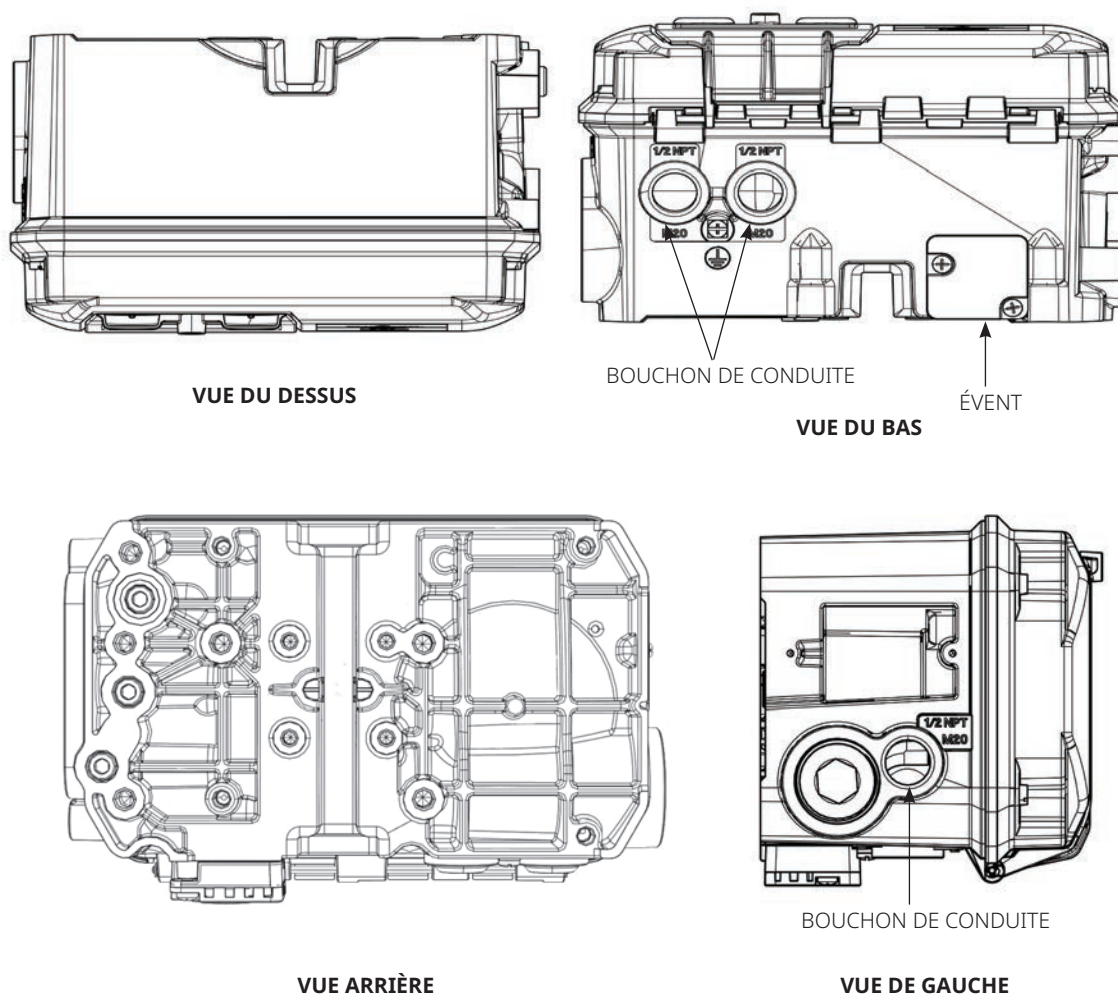
Figure 28. Schémas d'assemblage de l'appareil DVC7K (suite)
