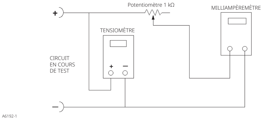
Figure 4. Schéma du test de tension
