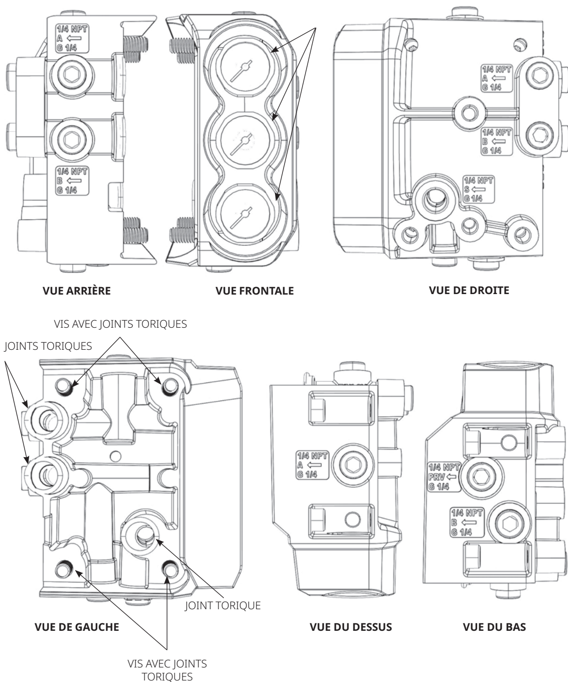
Figure 29. Ensemble manomètre
